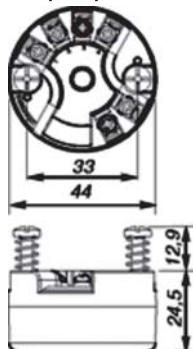
Измерительный преобразователь Метран-2700
