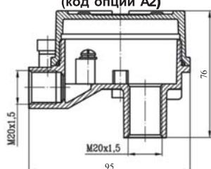
Соединительная головка (код опции A2)
