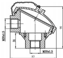
Соединительная головка (код опции A2)
