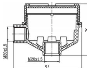
Соединительная головка (код опции P1)
