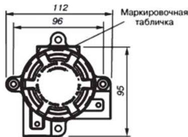
Универсальная головка (код опции A6)
