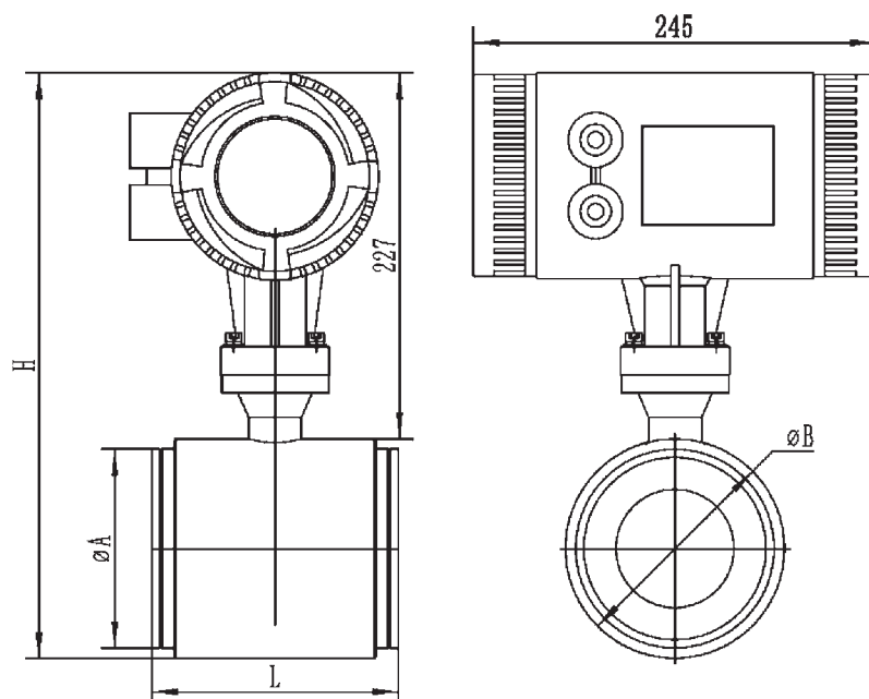
Рис. 20. Расходомер модели Метран-370MW с преобразователем интегрального монтажа.
