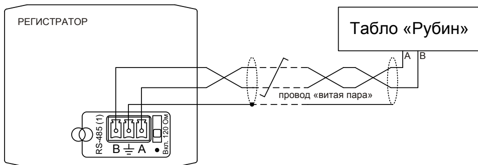
Рисунок Е.1 Подключение табло к регистратору по интерфейсу RS-485
