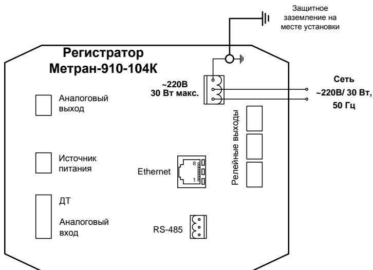
Рисунок Б.7 Подключение регистратора к сети питания
