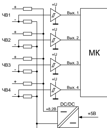
Рисунок 1.3. Структурная схема группы из 4-х частотно-импульсных входов
