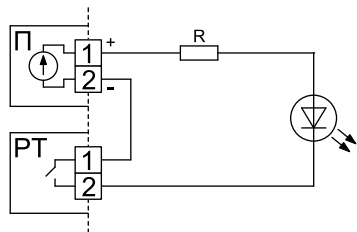
Рисунок Б.4 – Подключение выходов твердотельных реле (РТ).
