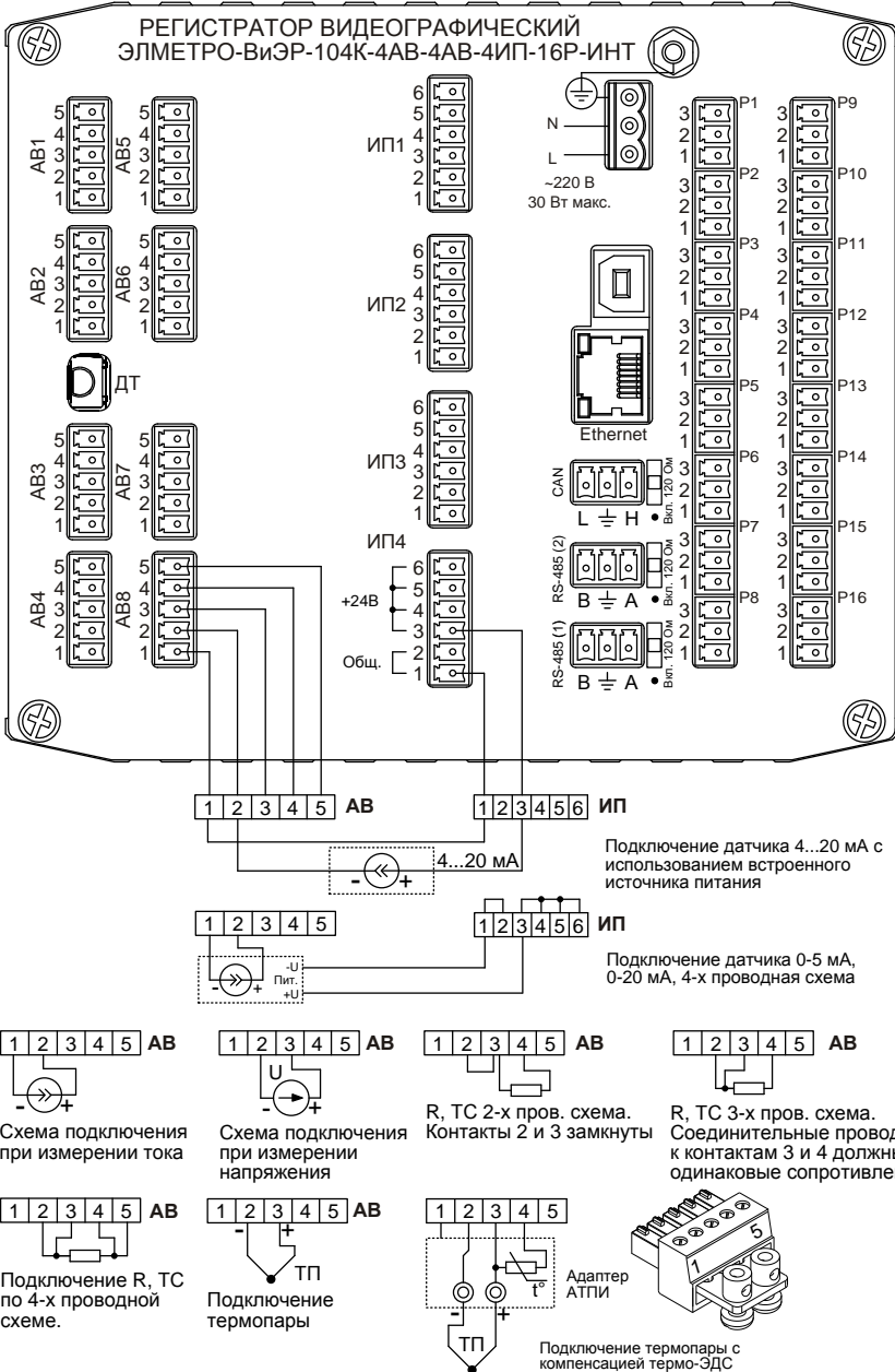
Рисунок Б.1 – Подключение датчиков к каналам АВ.
