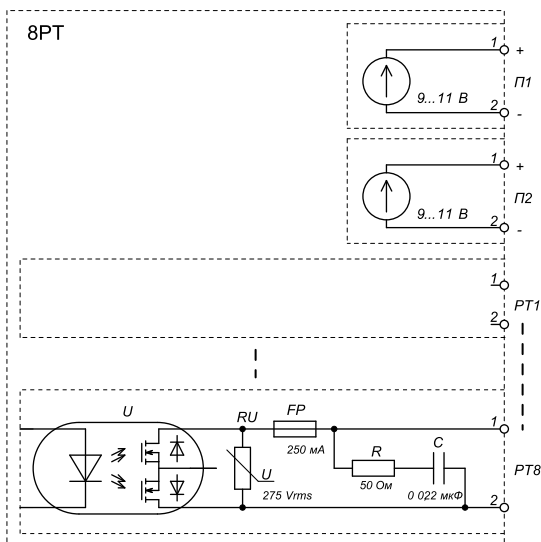
Рисунок 1.2 Устройство платы 8РТ
