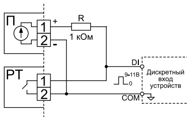
Рисунок Б.4 – Подключение выходов твердотельных реле (РТ).
