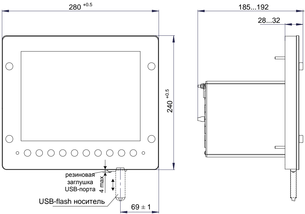
Рисунок А.1 Габаритные размеры регистратора
