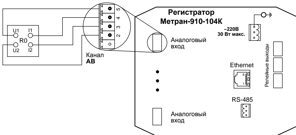
Схема подключения при измерении сопротивления и сигналов ТС каналами АВ
