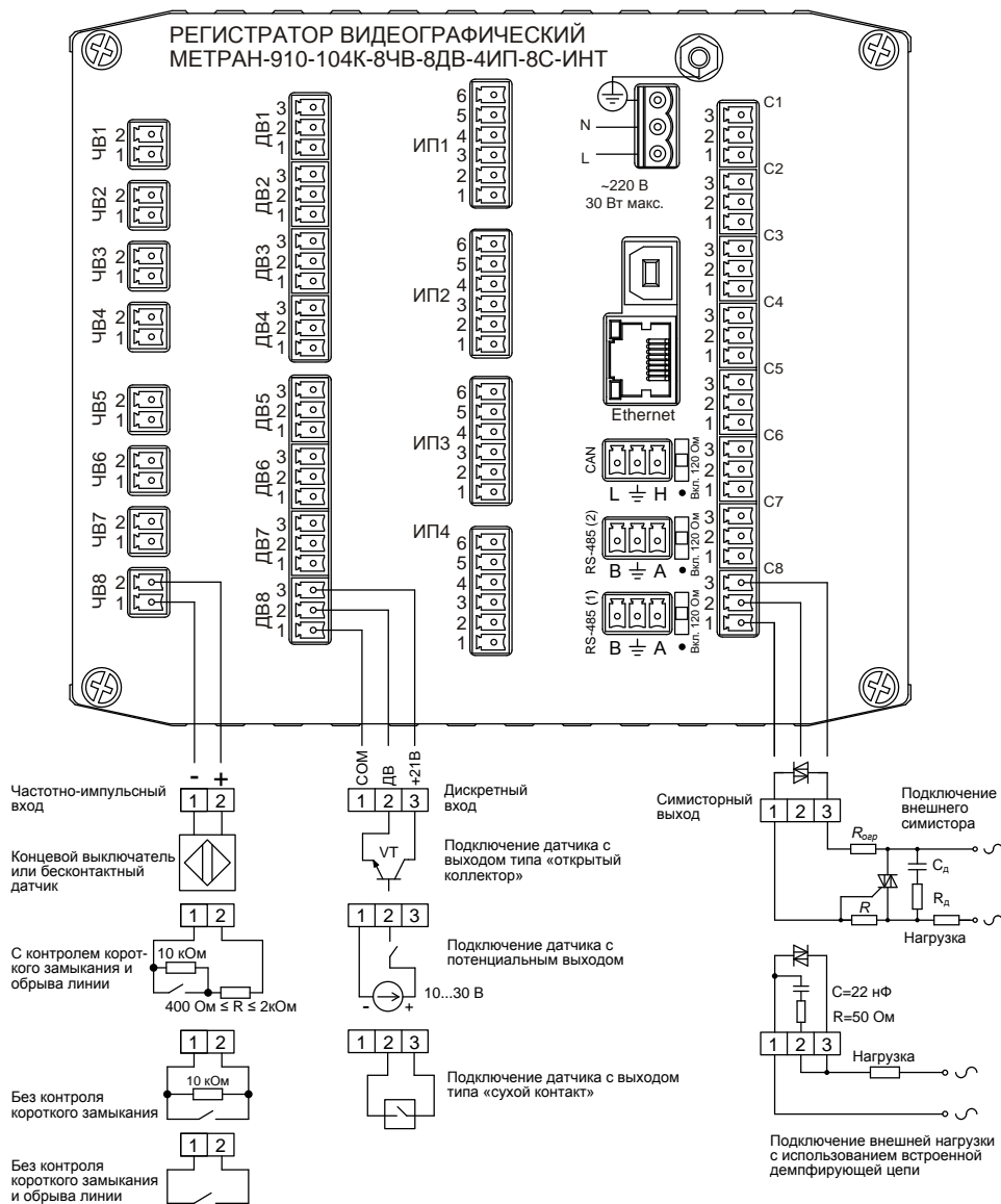
Рисунок Б.3 – Подключение дискретных/частотных входов и симисторных выходов.
