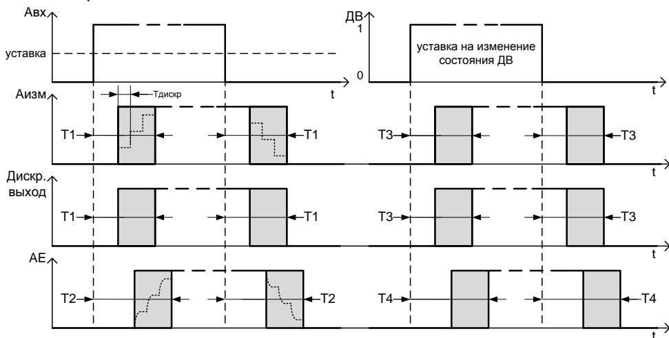
Рисунок 1.4. Временная диаграмма, описывающая реакцию цепей сигнализации T_{дискр} = 0,1 с (внутренний цикл опроса каналов); Аизм – внутренняя переменная канала, результат измерения / вычисления (для ДВ – состояние), доступная к записи в архив прибора и к чтению через регистры Modbus , CAN; АЕ – значение тока на токовом выходе АЕ
