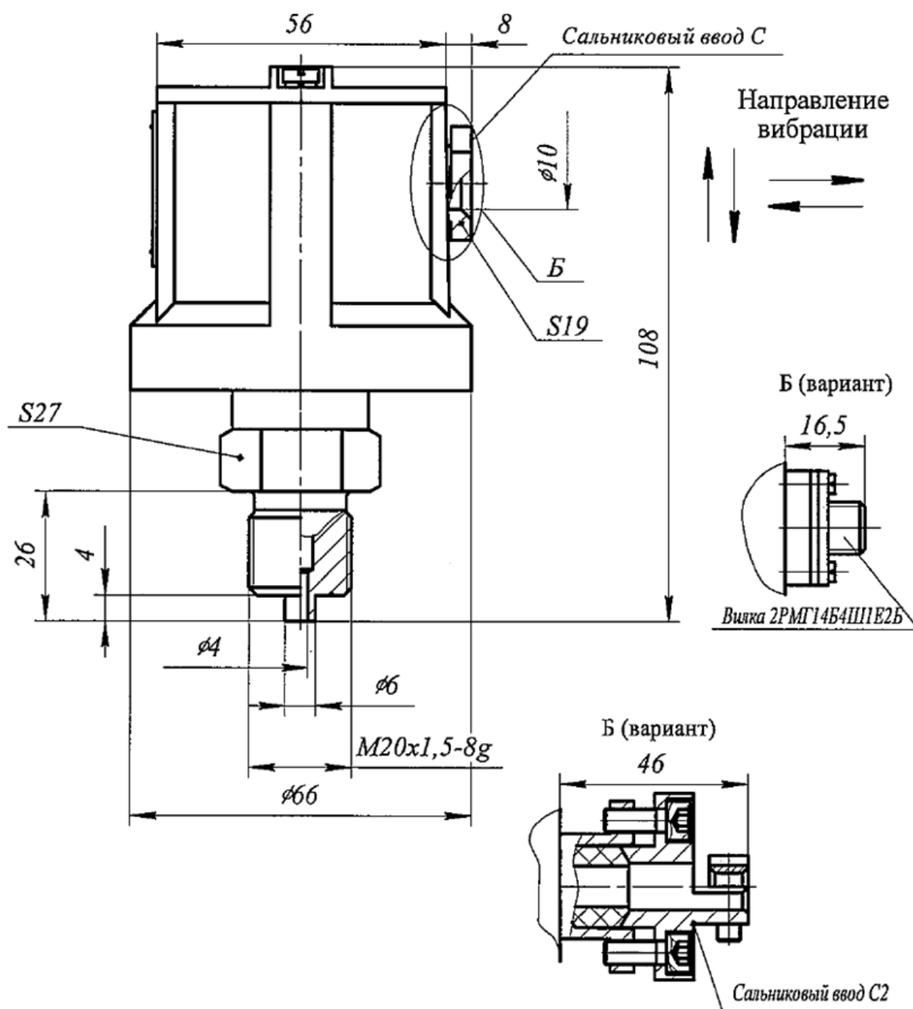
Рисунок Д.1 - Метран-55 модели 515, 516, 517, 518, 528, 535.
