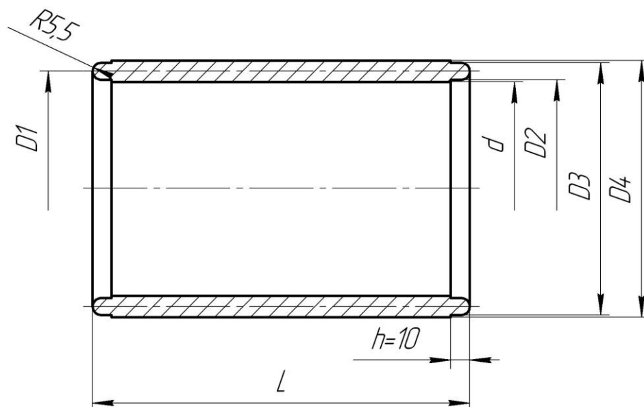
Рисунок Ж.1 – Технологическая вставка
