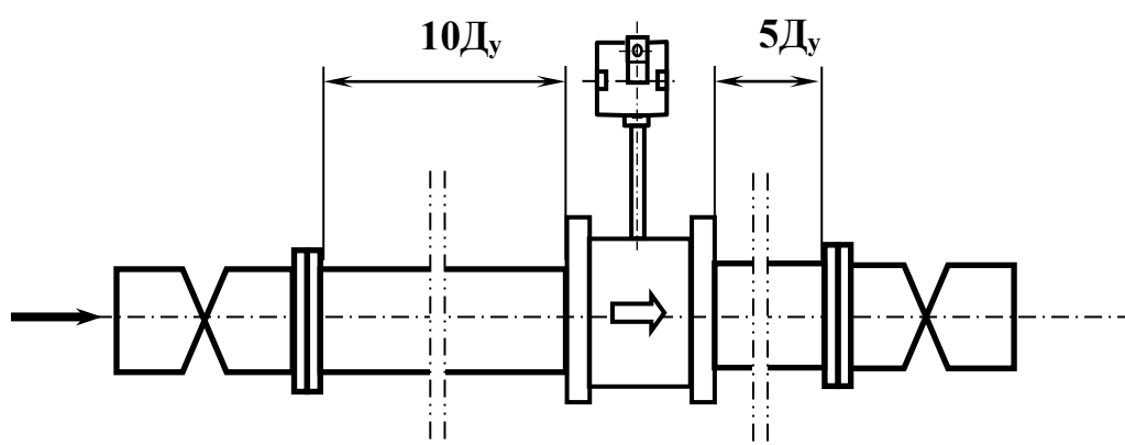
Рисунок Е. 7 - Установка преобразователя с двумя дроссельными клапанами
