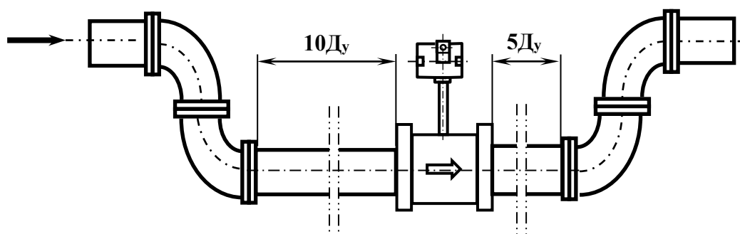
Рисунок Е.5 - Установка преобразователя с двумя отводами 90^\circ в одной плоскости
