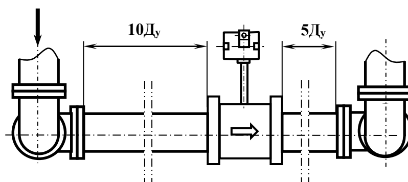
Рисунок Е. 6 - Установка преобразователя с двумя отводами 90^\circ в различных плоскостях
