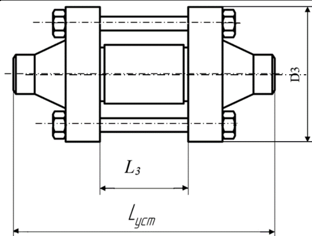
Рисунок Д.2 – Преобразователь с фланцами
